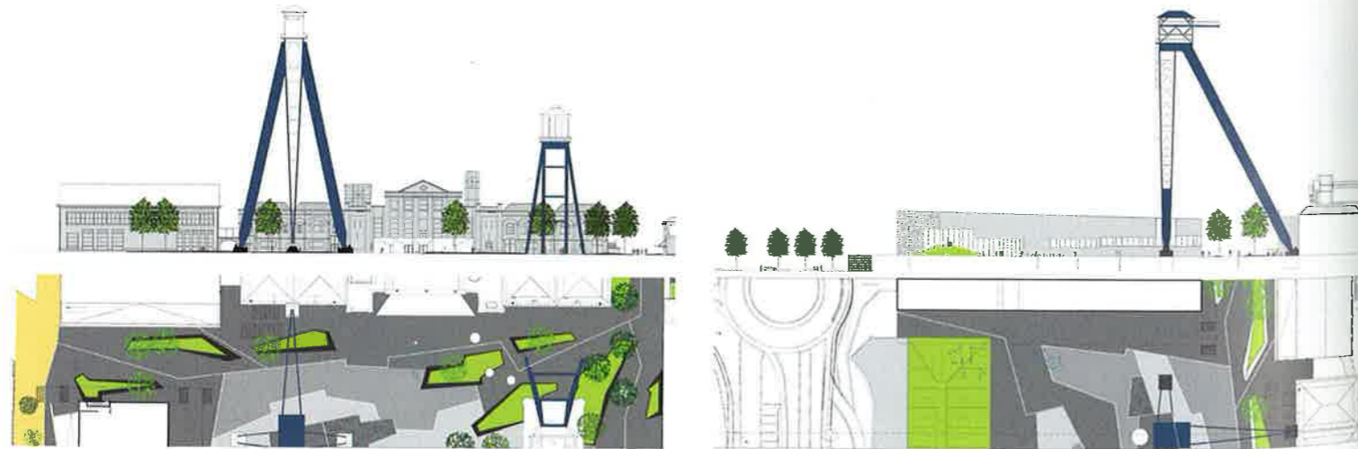
Plankaart, doorsneden en plattegronden met daarop onder meer de nieuwe en bestaande bomen, ledverlichting in het plein en de over het plein 'gestrooide' rode stalen stoelen.
